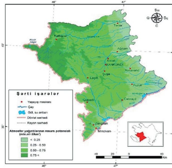
Şəkil 3. Qarabağda atmosfer yağıntılarının resurs potensialı xəritəsi
