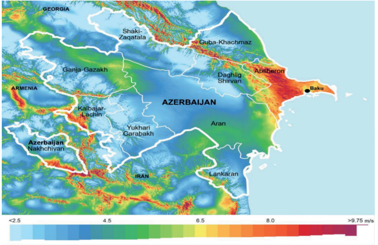
Şəkil 2. Azərbaycanda külək enerjisi potensialı. ( Mənbə: Dünya Bankı)
