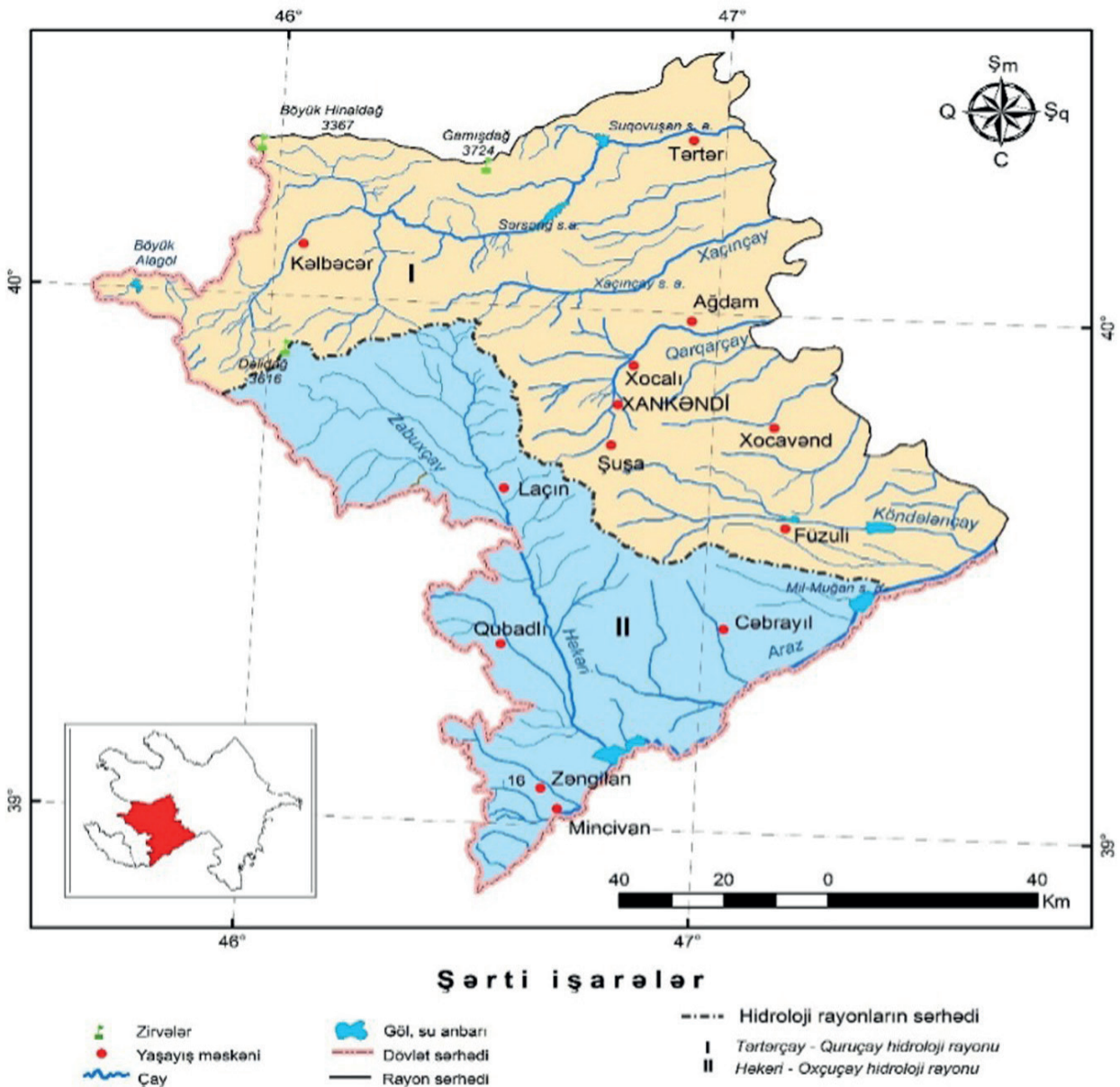
Şəkil 2. Qarabağda axımın hündürlükdən asılı olaraq dəyişməsinə əsasən hidroloji rayonlaşdırılması
