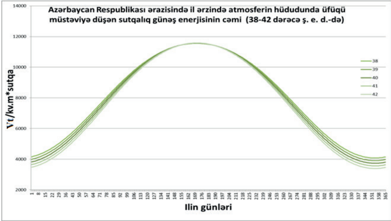
Şəkil 1. Günəş radiasiyasının qiymətləri
