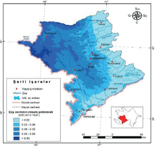
Şəkil 4. Qarabağda çay axımının resurs potensialı xəritəsi
